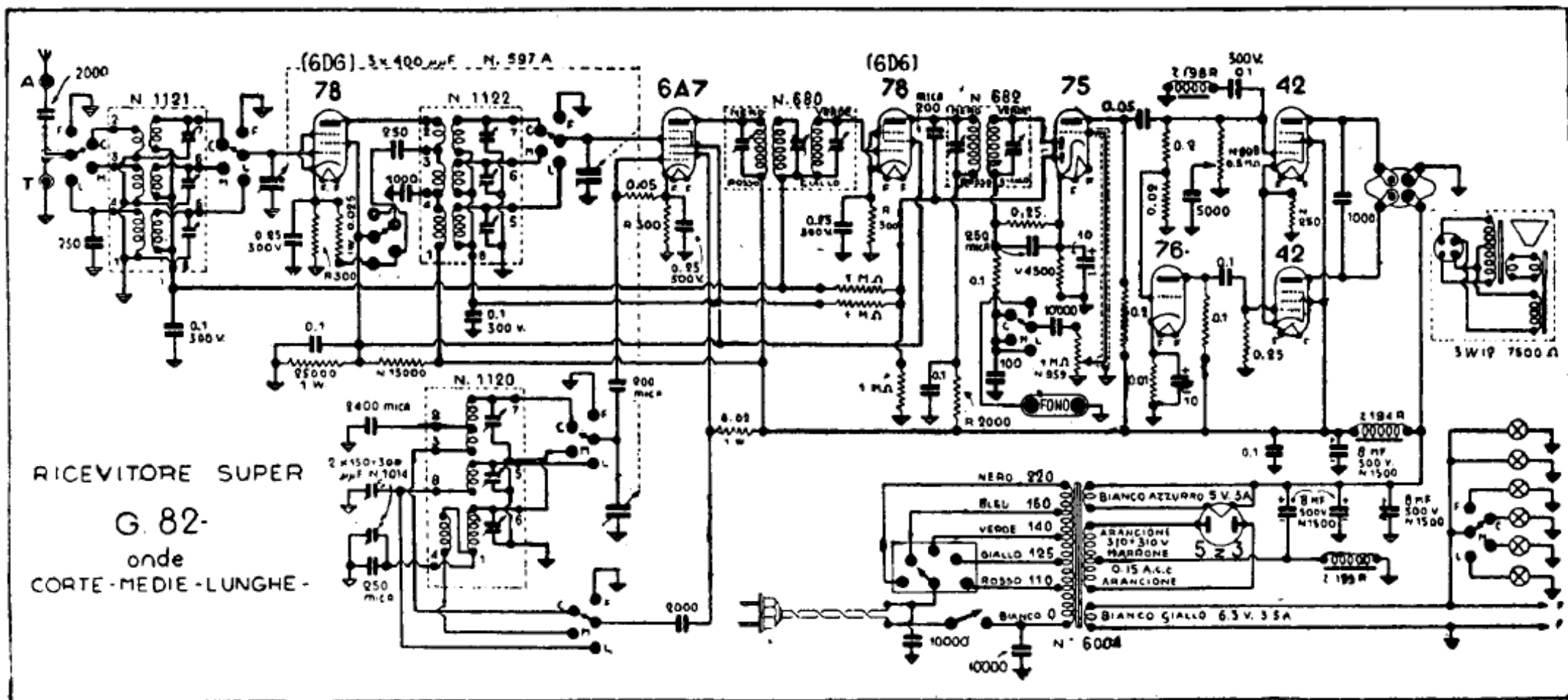
S. A. GELOSO. — Mod. G. 82. — 300 V al I° elettrolitico, 280 V al II°. — Media frequenza: 467 kHz. — Prod. 1937.
